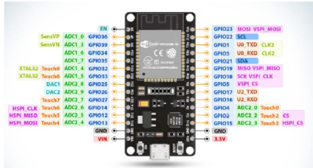
Fig. 3. ESP32 Dev Module
